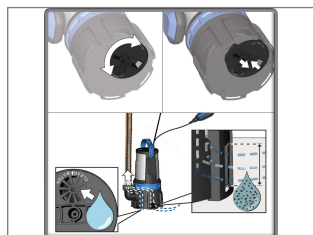
Ütésálló műanyagból készült szivattyúház
